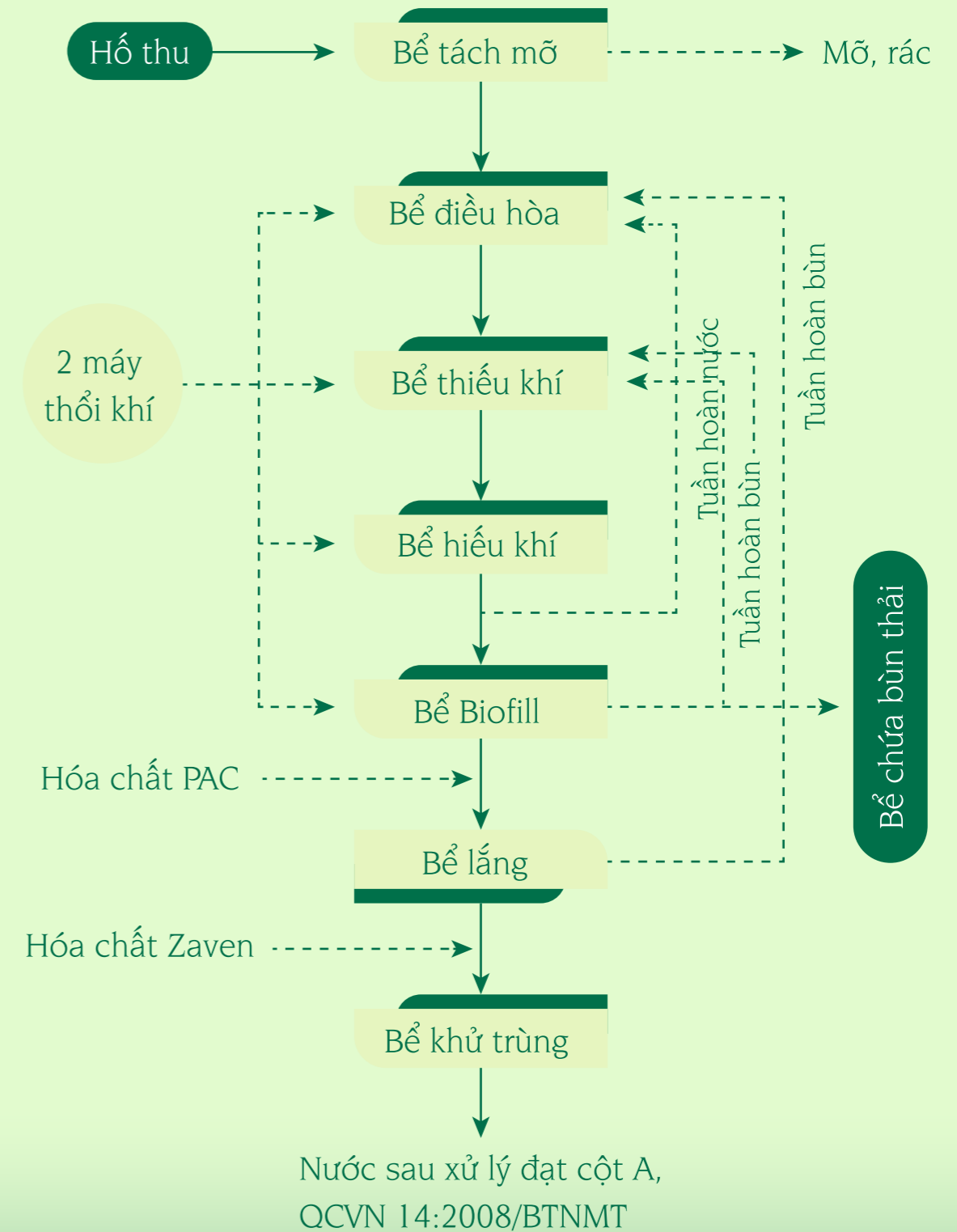
Sơ đồ quy trình công nghệ xử lý nước thải
